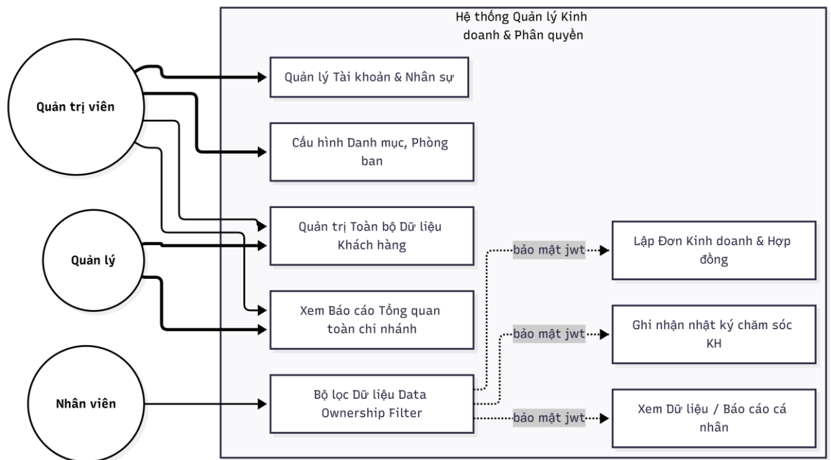
Hình 2.1. Sơ đồ minh họa phân quyền hệ thống
