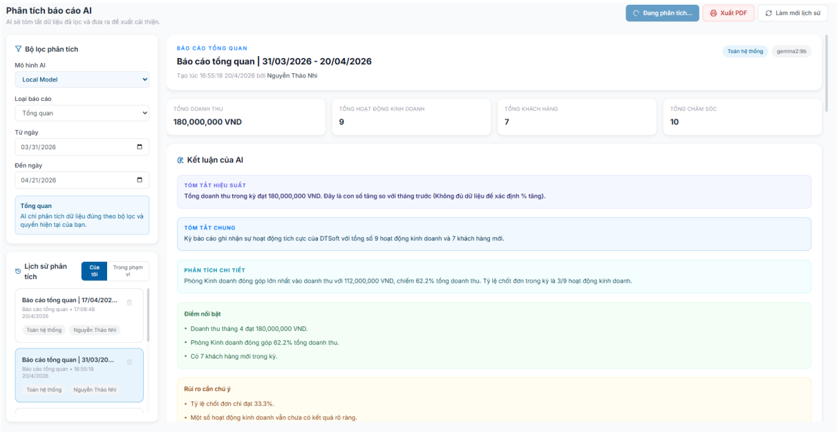
Hình 5.8. Chức năng AI hỗ trợ phân tích báo cáo thống kê
