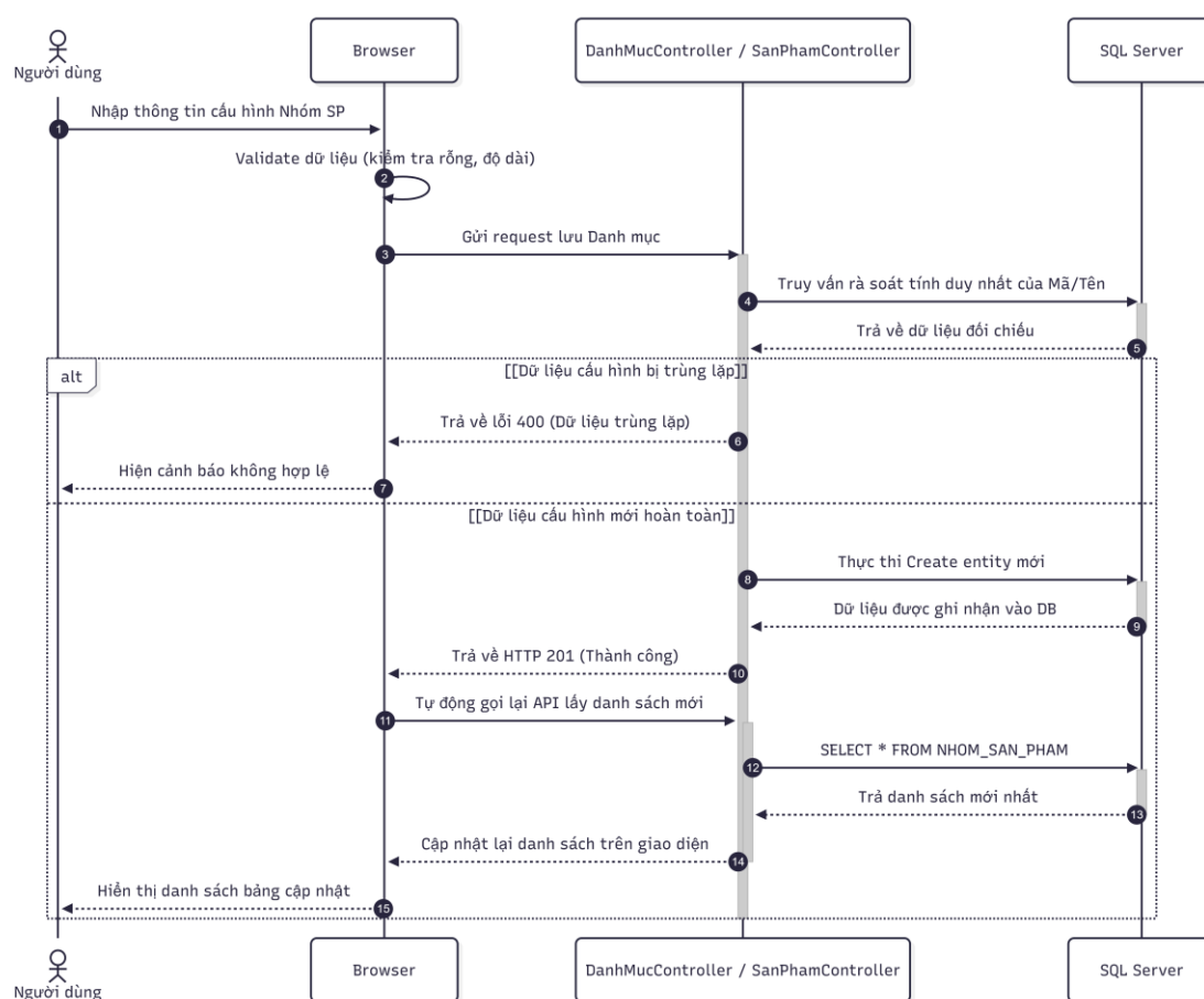
Hình 2.3. Biểu đồ tuần tự chức năng quản lý danh mục và sản phẩm
