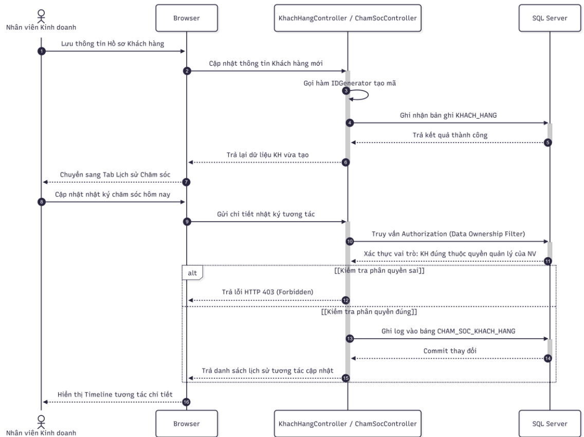
Hình 2.4. Biểu đồ tuần tự chức năng quản lý Khách hàng và Đối tác
