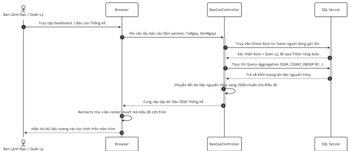
Hình 2.6. Biểu đồ tuần tự chức năng Báo cáo thống kê và Dashboard
