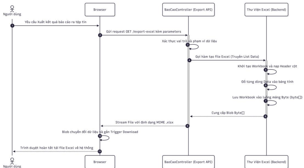
Hình 2.7. Biểu đồ tuần tự các chức năng mở rộng
