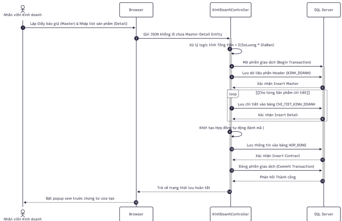
Hình 2.5. Biểu đồ tuần tự hoạt động Kinh doanh và Chứng từ
